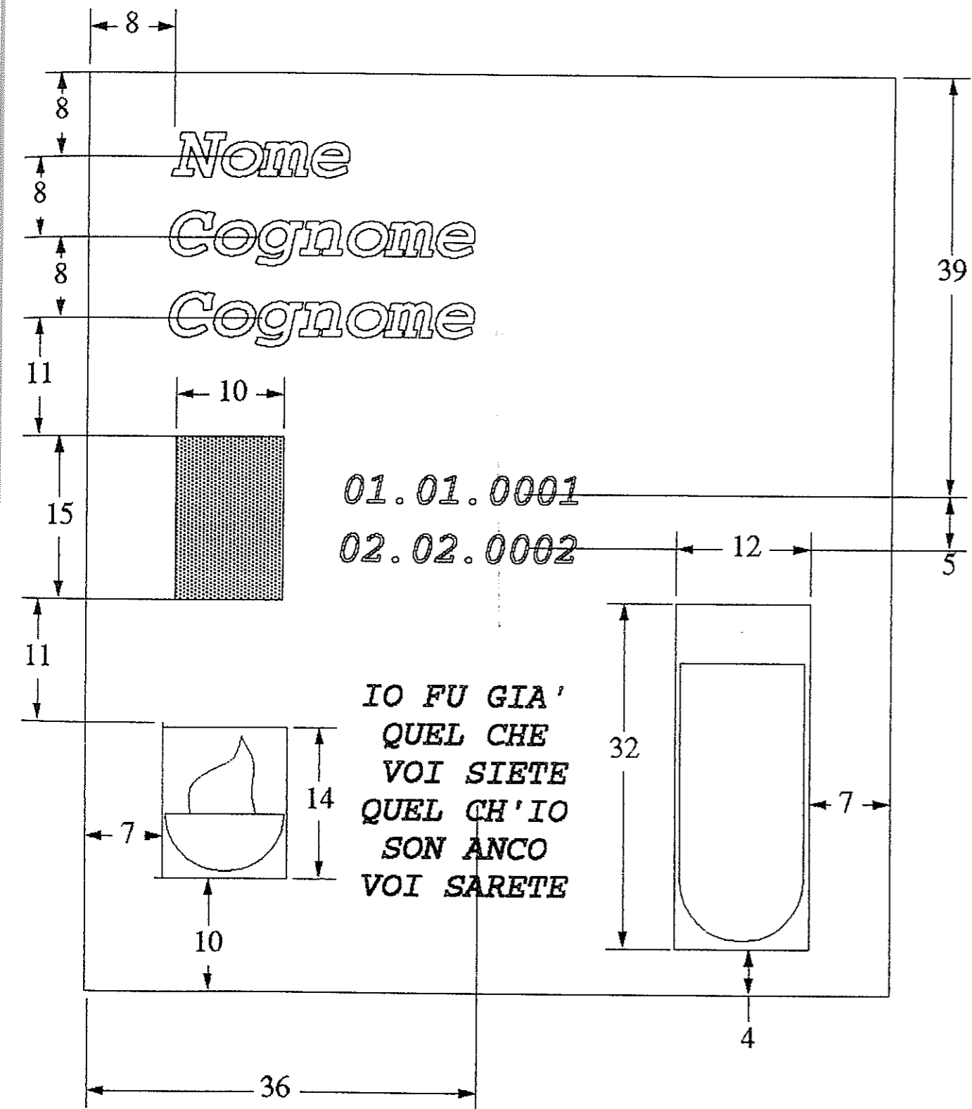
PARAMENTO 75X85 CM SCRITTA A BANDIERA (DESTRA) NOMI: BODONI (A/b) CORSIVO CONT. (OUTLINE) 50 MM NUMERI: BODONI CORSIVO CONT. (OUTLINE) 25 MM ISCRIZIONE: BODONI (A) CORSIVO CONT. (OUTLINE) 20 MM
