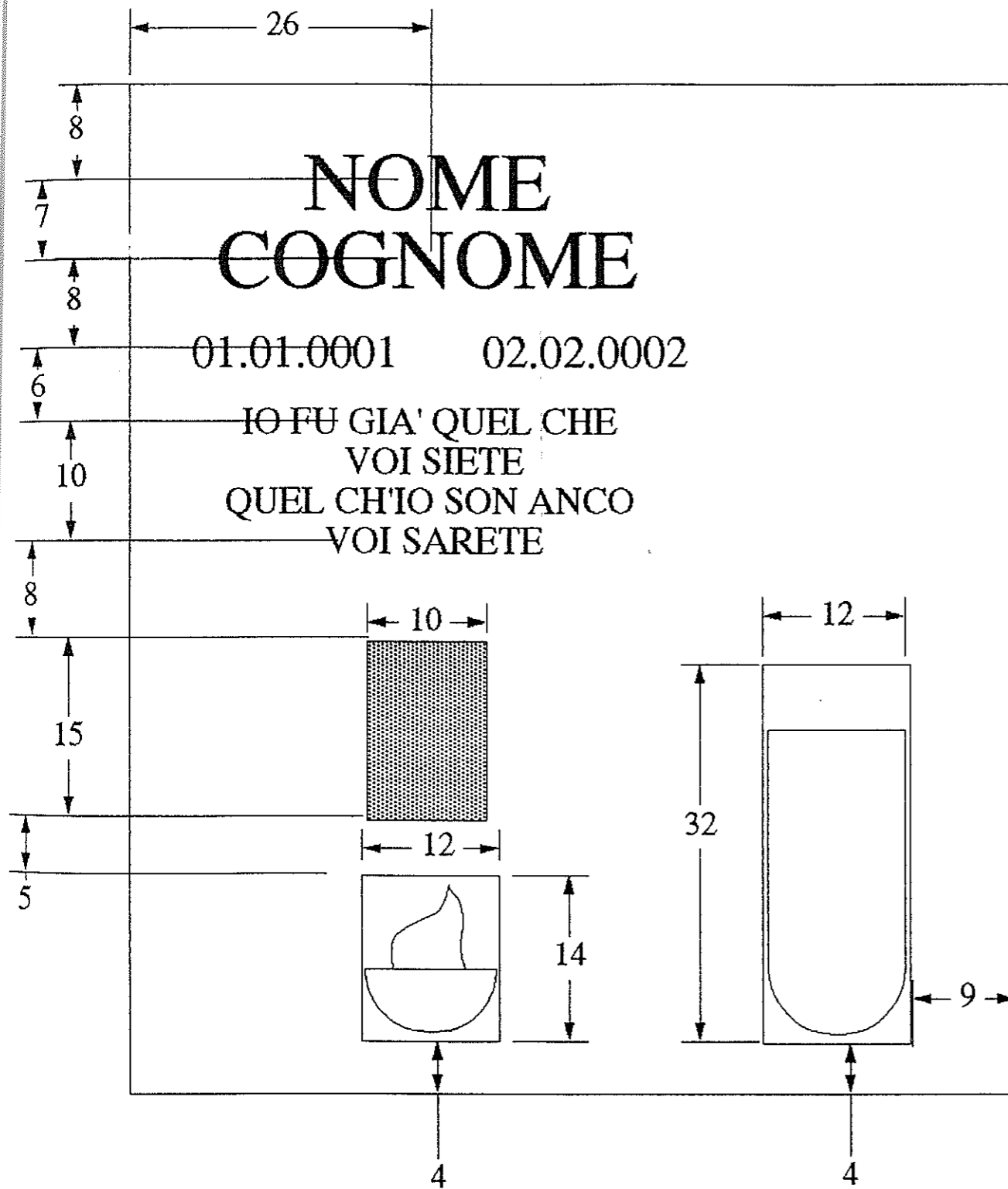
PARAMENTO 75X85 CM SCRITTA CENTRALE LAPIDARIA NOMI: BODONI (ALTO) LEGGERO (LIGHT) 50 MM NUMERI: BODONI LEGGERO (LIGHT) 25 MM ISCRIZIONE: BODONI (ALTO) LEGGERO (LIGHT) 20 MM
